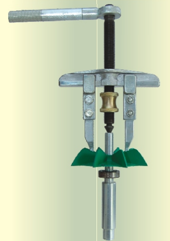
REMOVING MOTOR FAN
